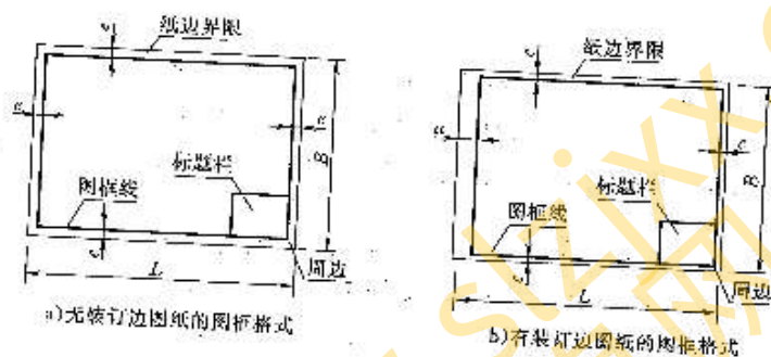
图 3.11.3-1 图框和标题栏
