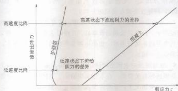
图1 泥浆与混凝土的流动性能关系
