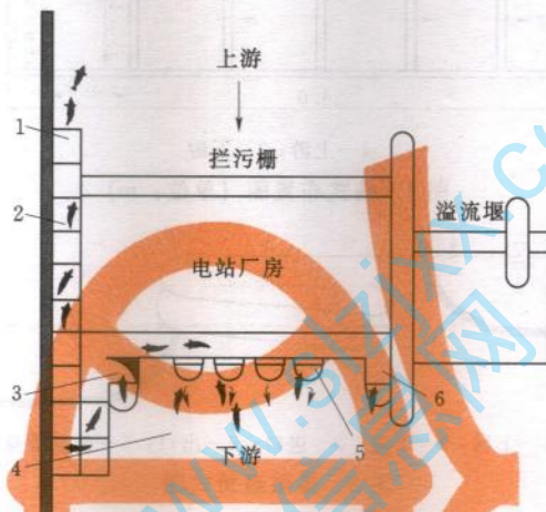
1—鱼道出口；2—鱼道槽身；3—鱼道进口；4—水流高紊动区； 5—集鱼系统进鱼口；6—集鱼系统水流出口（进鱼口）
