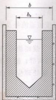
图 6.3.2 槽式鱼道横断面示意图
