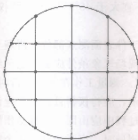
图 2 圆形平面测点布置示例图
