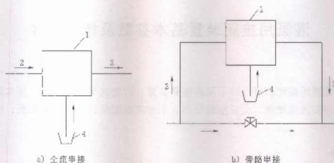
图1 串接水动式施肥泵示意图
