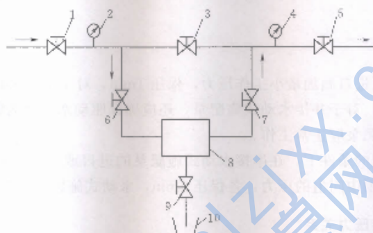
1、3、5、6、7、9—阀门；2、4—压力表； 8—比例式施肥泵；10—喷嘴
