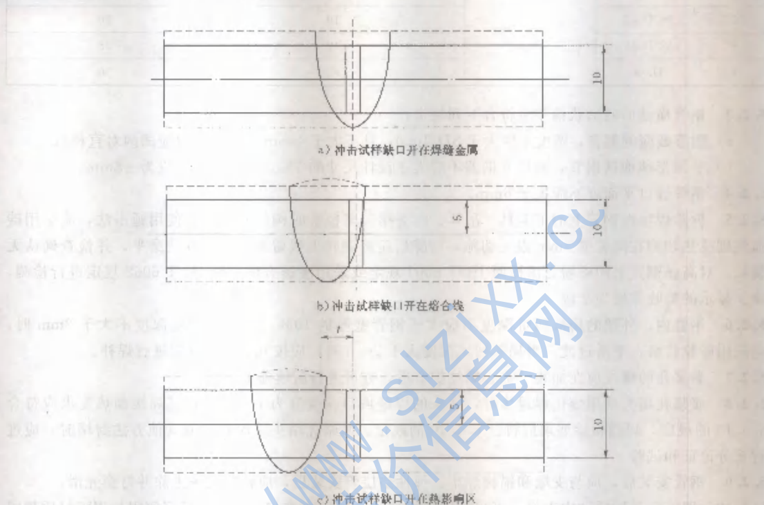
图 1 焊接接头冲击试样缺口位置图
