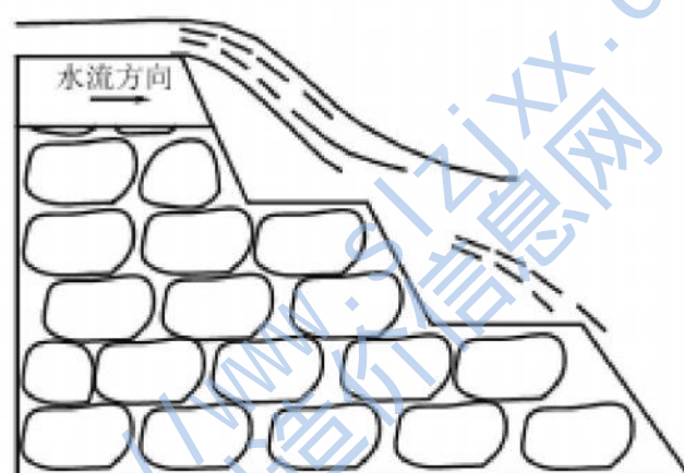
(d) 纵剖面图
