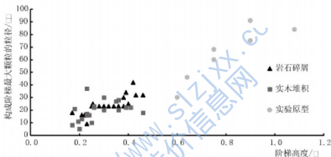
图 9 阶梯-深潭系统中的阶梯高度与构成阶梯的粒径间的关系
