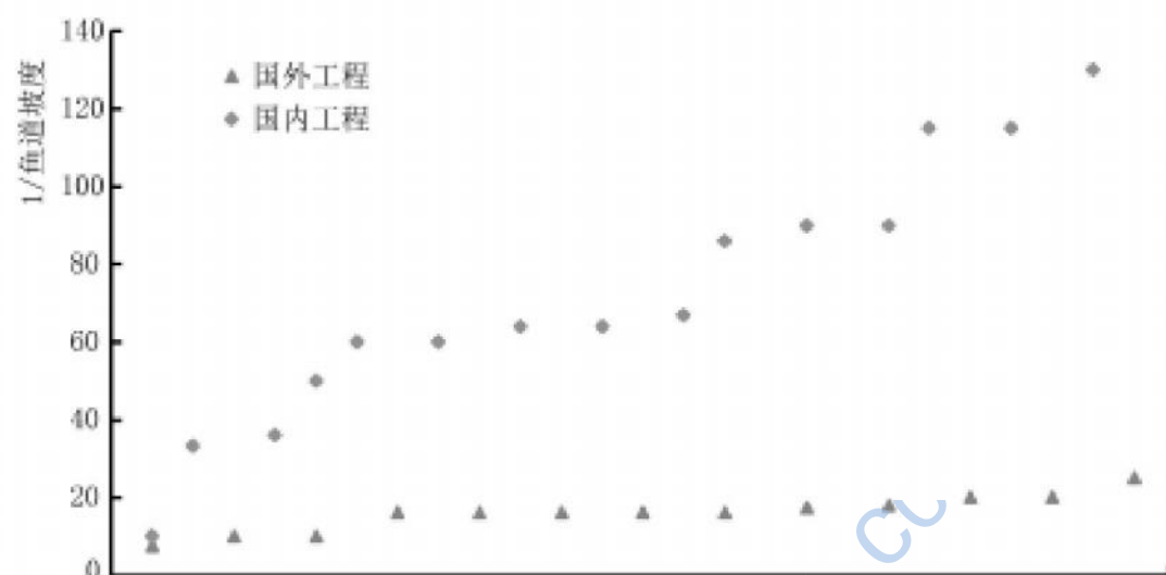
图 5 国内外部分鱼道坡度
