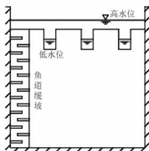
(c) 横剖面图
