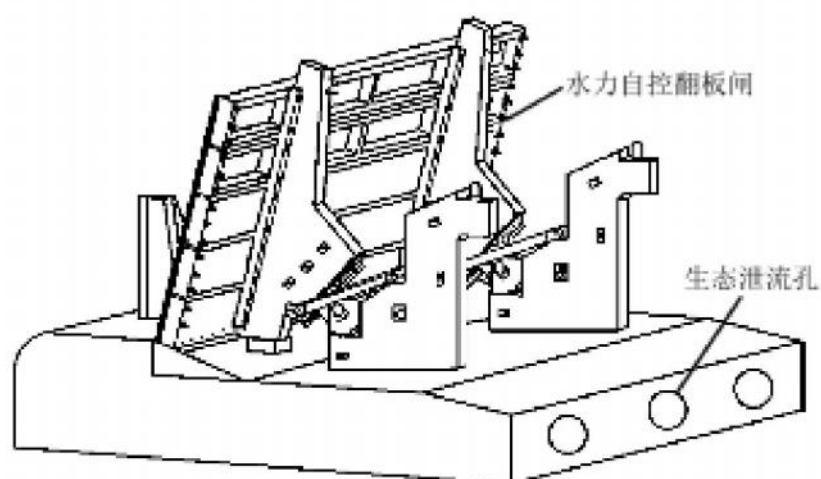
图7 底部基础带生态泄流孔的水力自控翻板闸结构示意图
