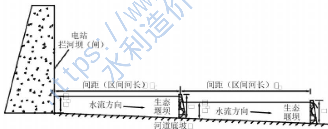
图 6 生态堰坝的高度及间距关系示意图
