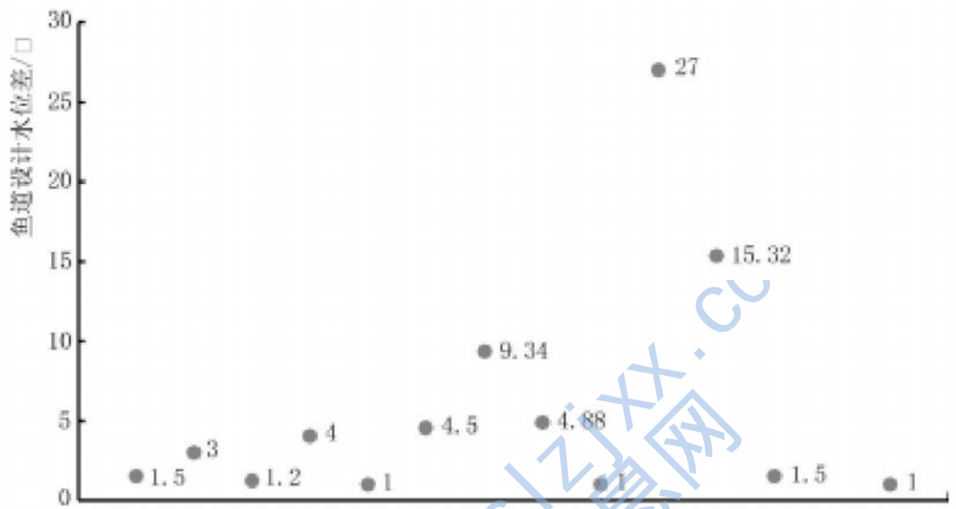
图 4 我国部分鱼道设计的水位差
