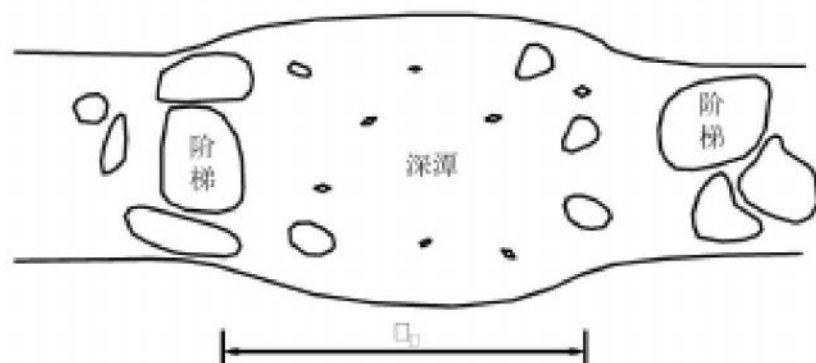
(b) 阶梯-深潭多级效能系统俯视图
