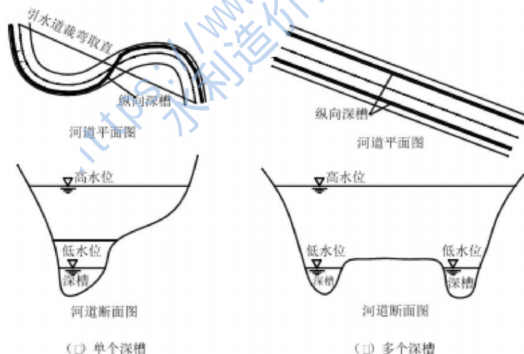
图 11 河道纵向深槽示意图
