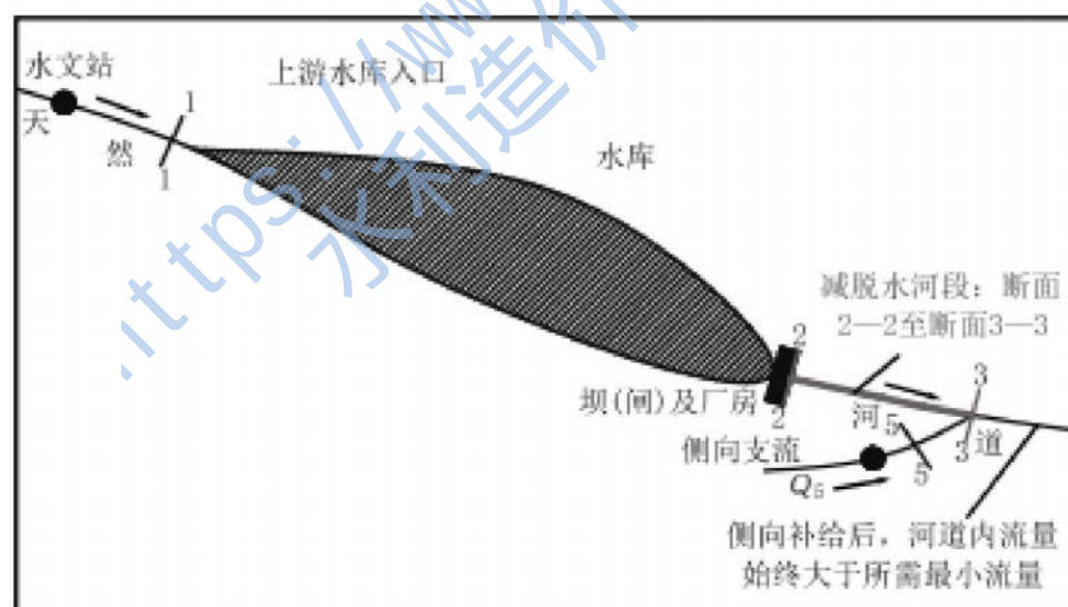
(E) 坝式水电站减脱水河段示意图
