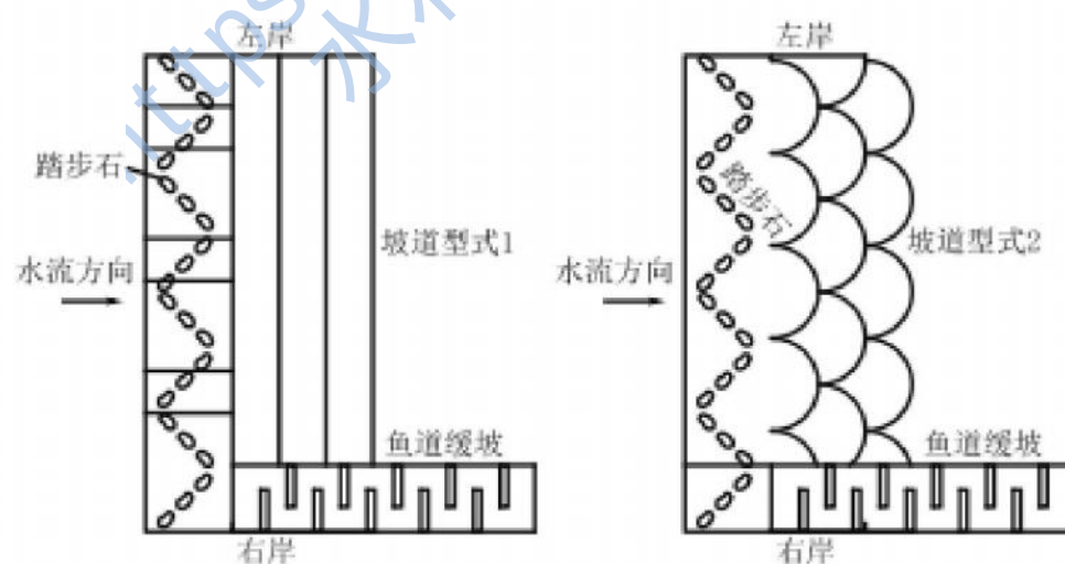
(e) 平面图
