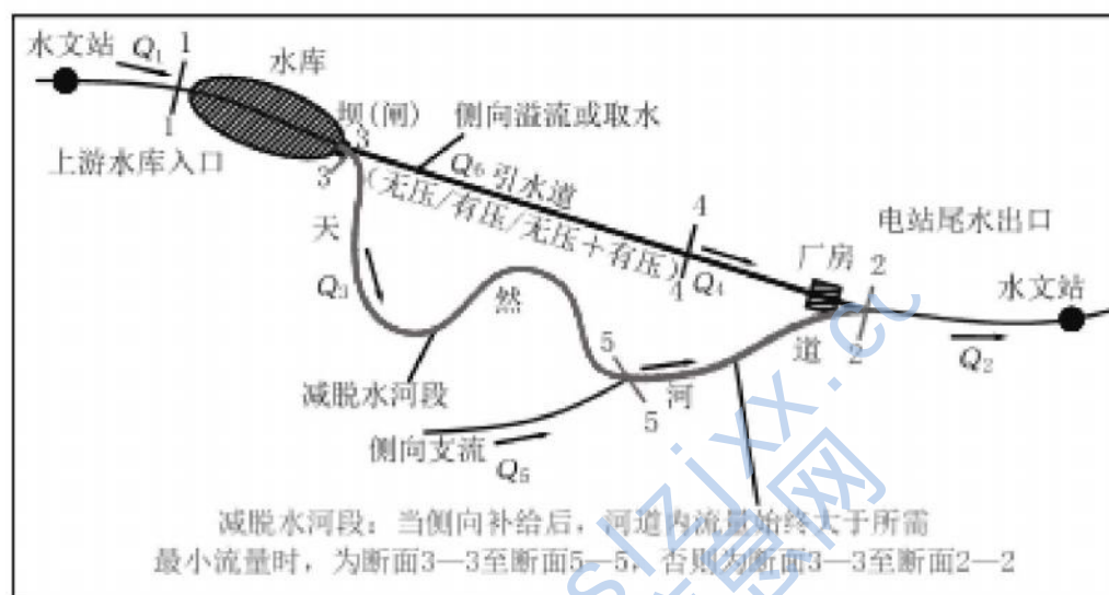
(D) 引水式、混合式水电站减脱水河段示意图
