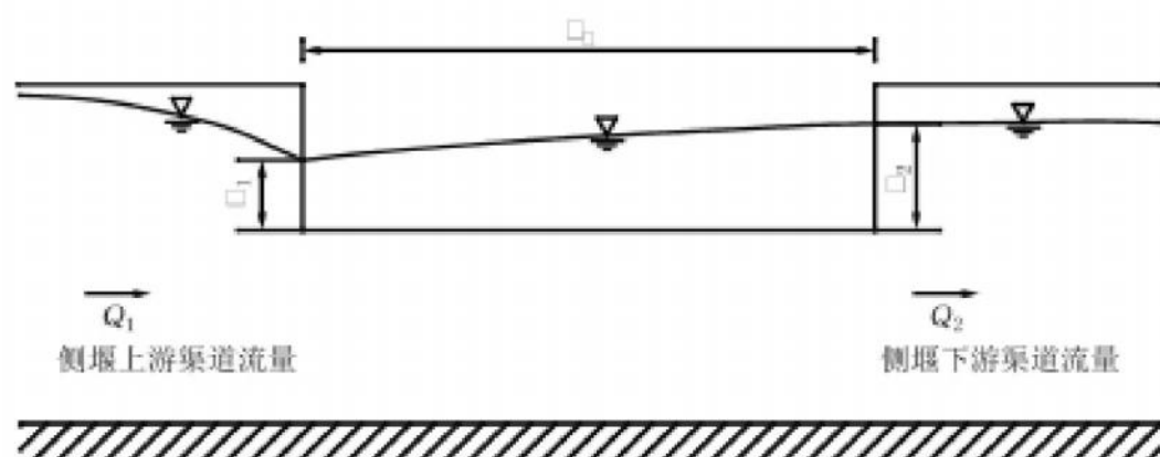
图 A.0.2 无压生态泄流孔（槽）矩形断面侧堰泄流计算简图
