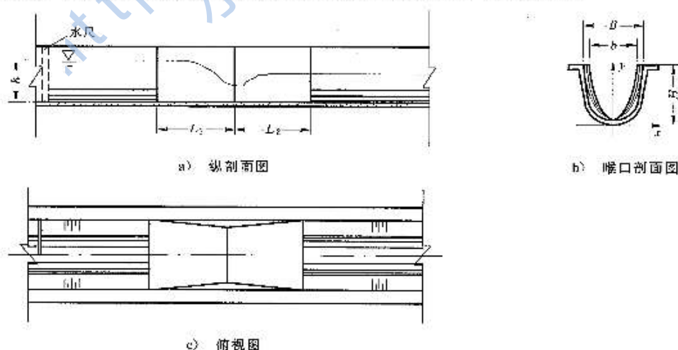
图 17 抛物线形喉口量水槽示意图
