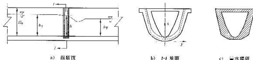
图 11 抛物线形移动式量水堰板的构造
