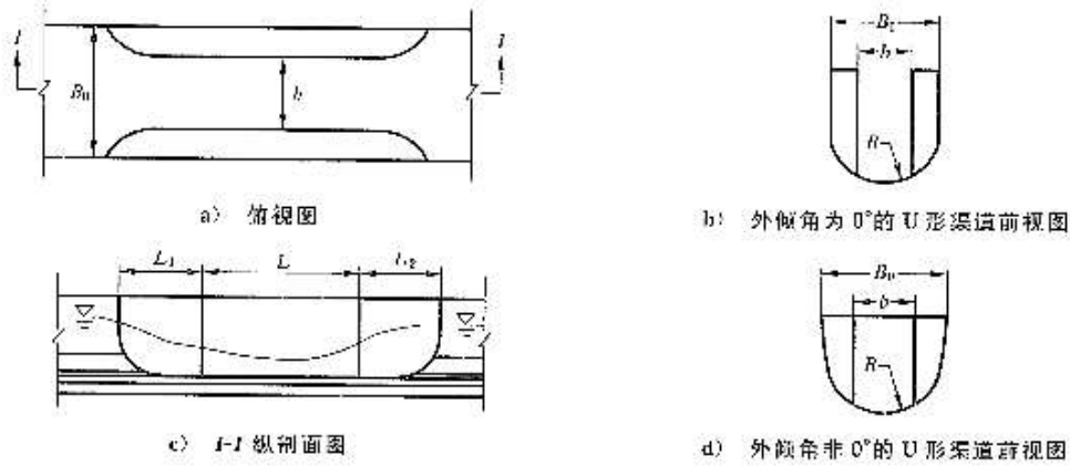
图 18 直壁式量水槽结构图
