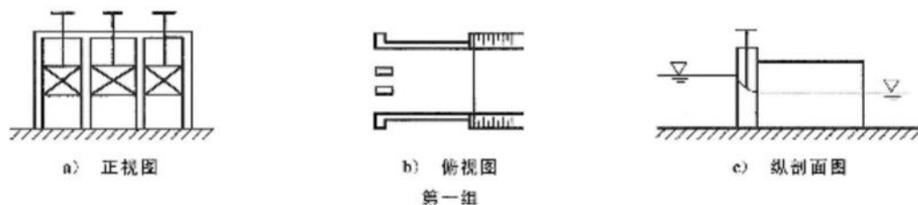
图5 明渠矩形直立式多孔平板闸示意图
