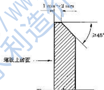
图 7 薄壁堰堰口锐缘加工图
