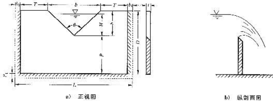
图 8 三角形薄壁堰示意图
