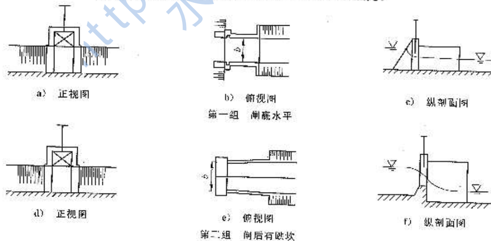
图 2 明渠直立单孔平板闸示意图
