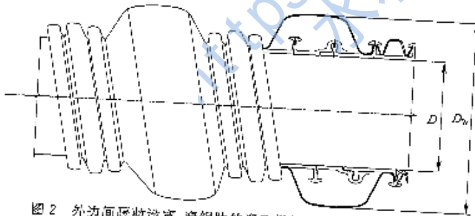
图2 外边间隔设置宽、窄钢筋的聚乙烯钢筋螺旋复合管材示意
