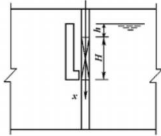
图E.0.1 快速闸门下落运动
