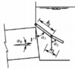
图C.0.2 双节式拍门开启角
