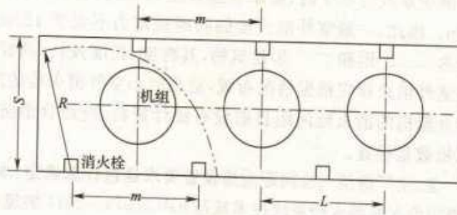
图2 消火栓交叉布置
