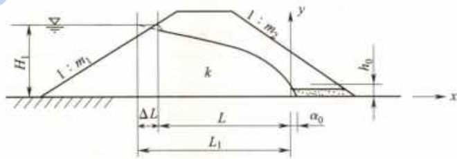
图 E. 2.2 有褥垫式排水土堤计算
