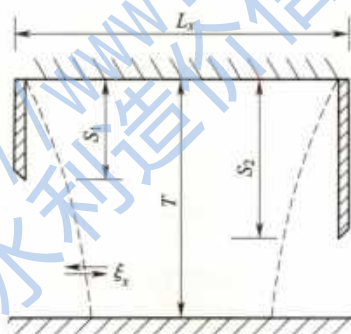
图 E. 8. 3-3 水平段
