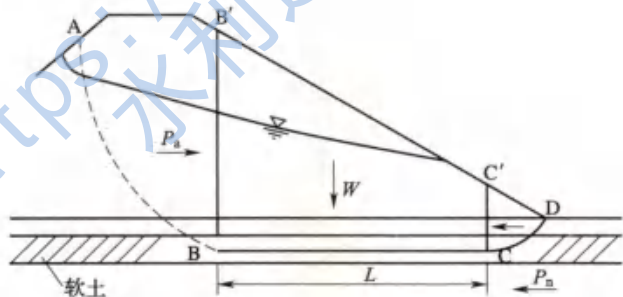
图 F.0.5 改良圆弧法计算
