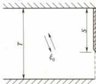
图 E. 8. 3-1 进、出口段
