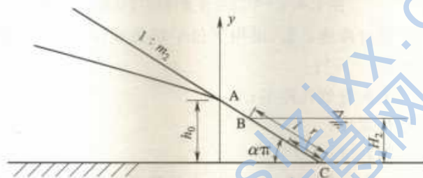
图 E. 5.1-2 下游有水计算( \alpha \pi 以弧度角计)
