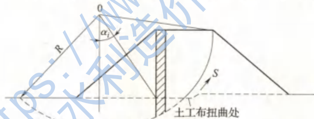
图 2 荷兰计算模型
