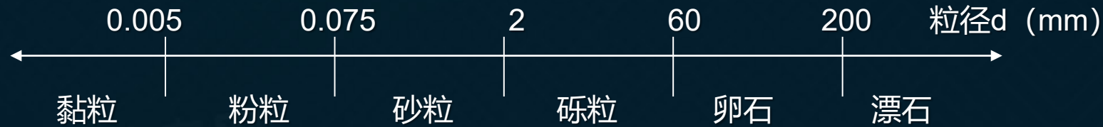
图1-1-1 土的粒径分组
