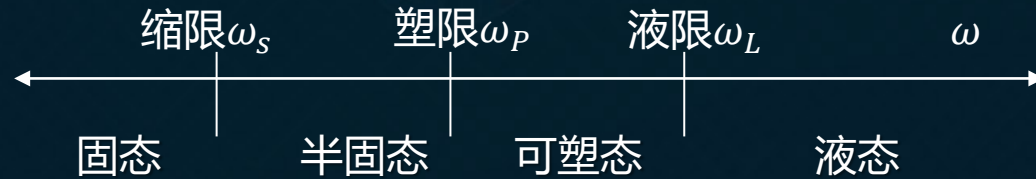
图1-1-2 土的稠度状态及界限含水率
