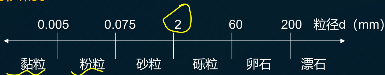
图1-1-1 土的粒径分组
