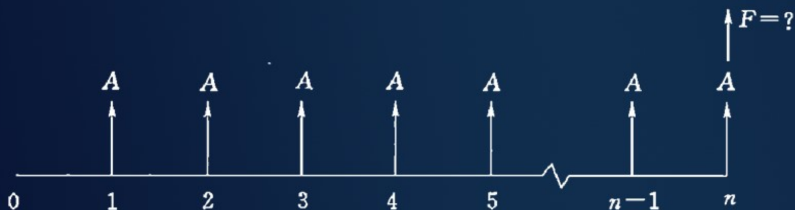
图2-1-5 等额年金终值公式现金流量图
