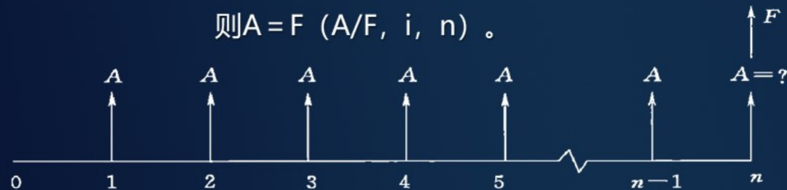
图2-1-7 偿债基金公式现金流量图
