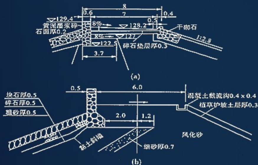
图 3-3-20 典型坝顶构造图 (单位:m)
