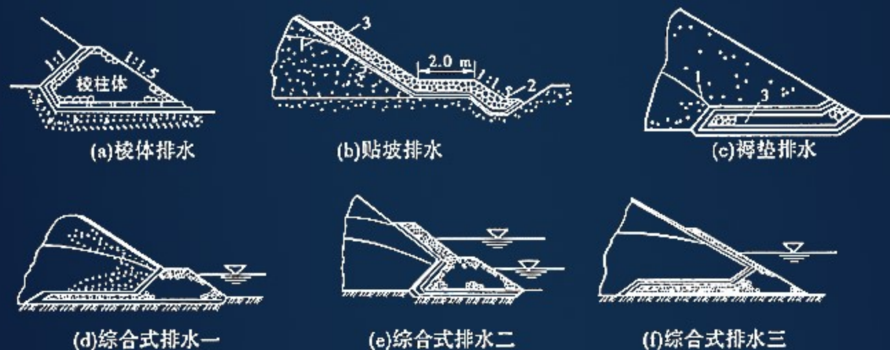
图 3-3-19 土石坝坝体排水设施主要型式
