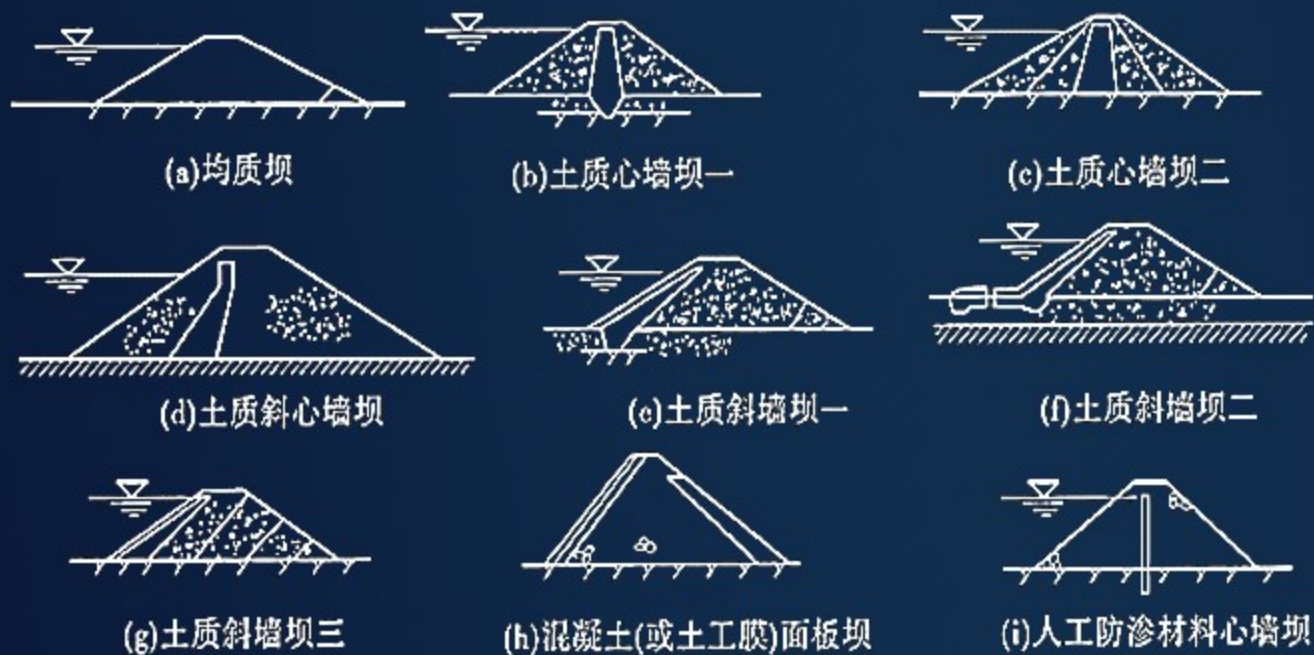
图 3-3-12 碾压式土石坝的类型
