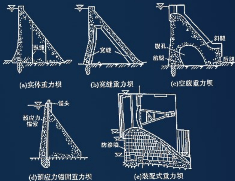
图 3-3-2 重力坝的型式
