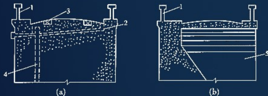
1—挡浪墙;2—坝顶排水管;3—起重机轨道;4—坝身排水;5—拱桥结构
