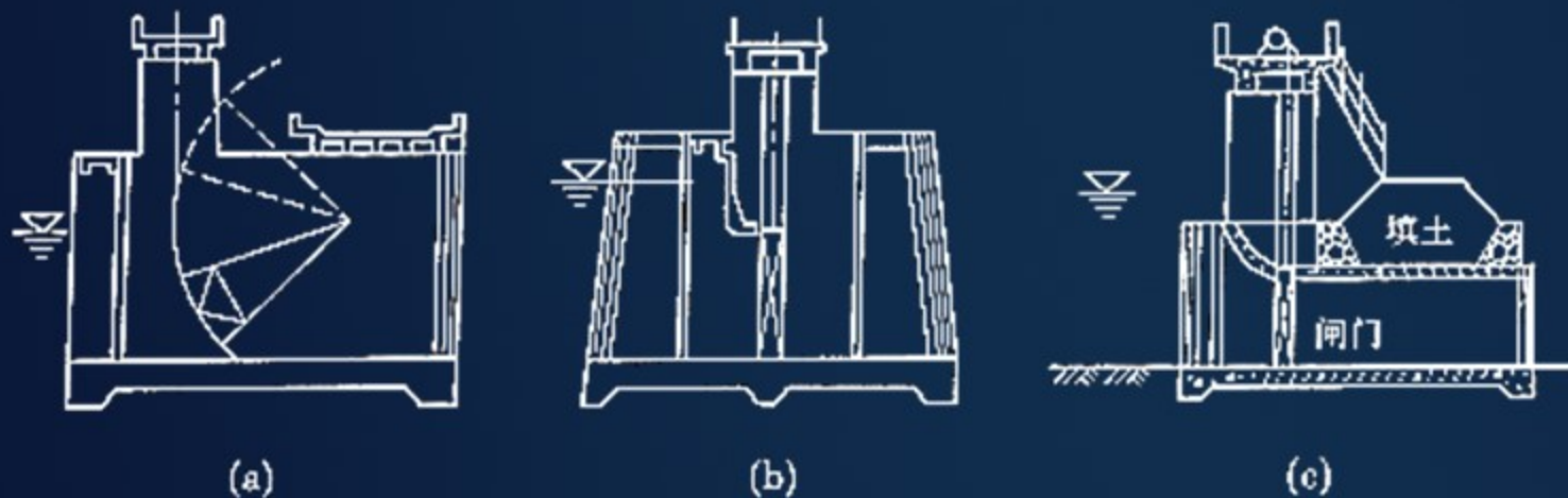
图 3-4-3 水闸的结构型式
