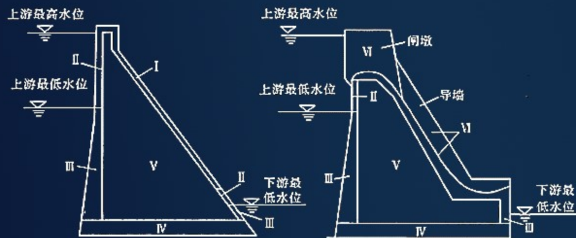
图 3-3-4 坝体混凝土分区图
