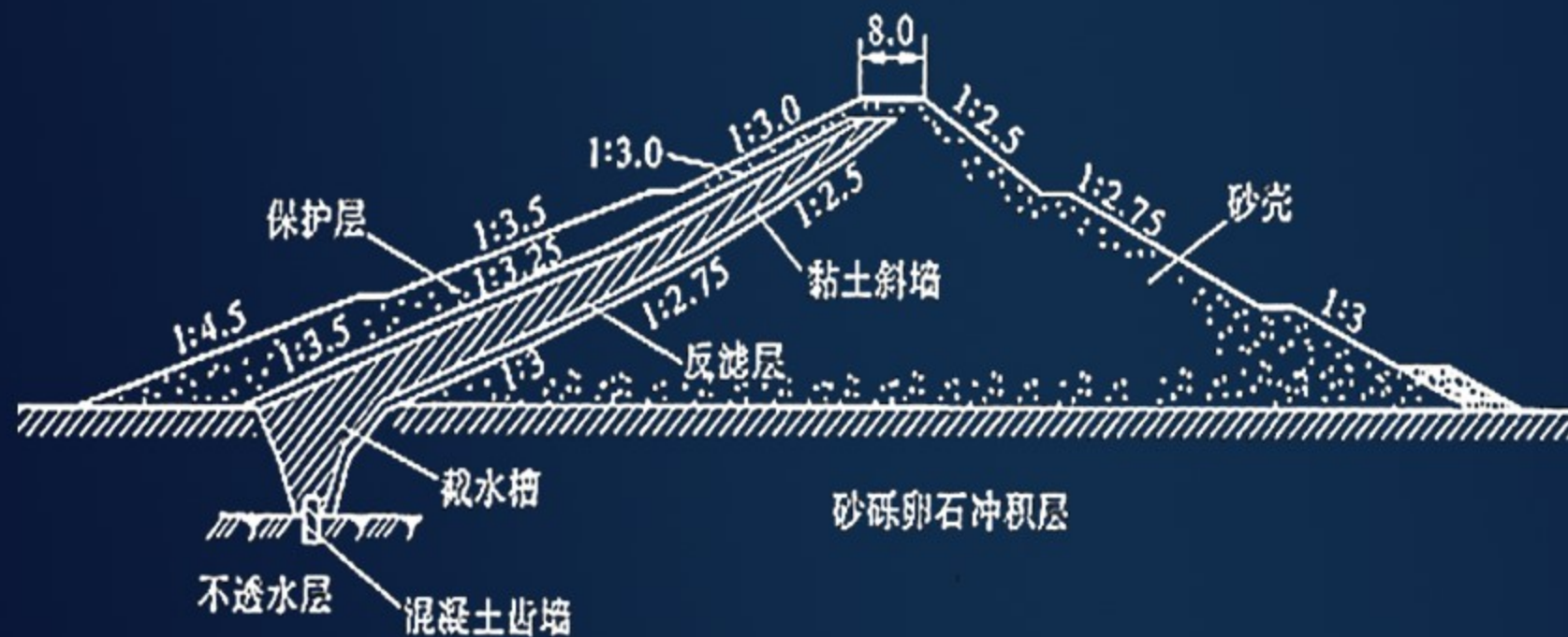
图 3-3-14 黏土斜墙坝 (单位:m)
