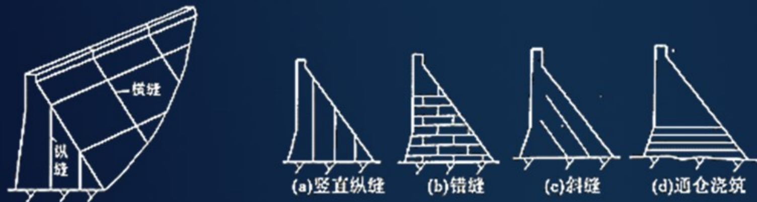
图 3-3-6 重力坝的横缝及纵缝
