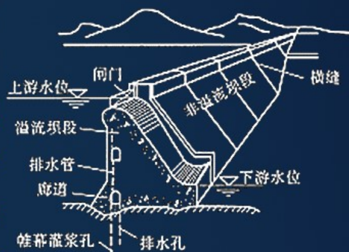
图 3-3-1 混凝土重力坝示意图
