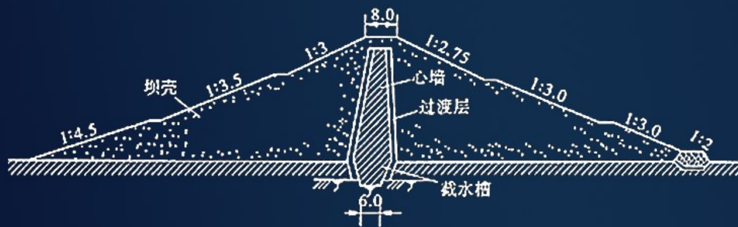
图 3-3-13 黏土心墙坝 (单位:m)
