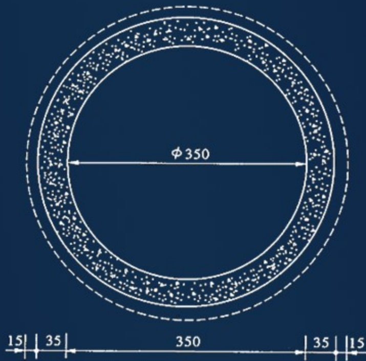
图 3-1 引水隧洞断面（单位：cm）
